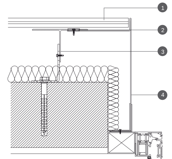
Detalle Jamba Metálica Metalic Jamb Detail
