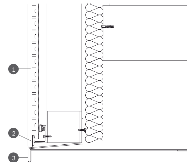
Detalle Dintel Metálico Metalic Lintel Detail
