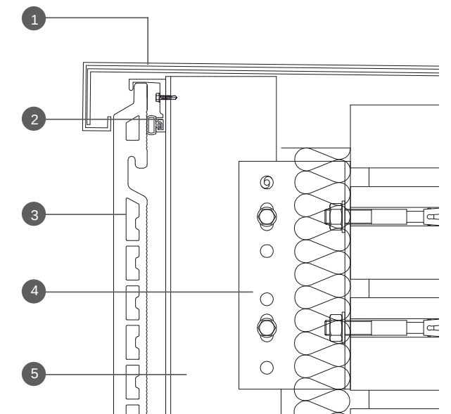
Detalle de coronación Coping Details
