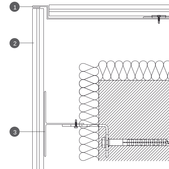
Detalle Esquina de Tapa Top Corner Detail
