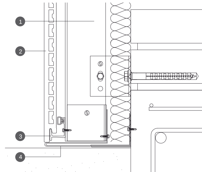
Detalle de arranque Base Details
